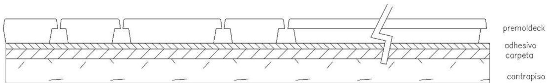
Corte-detalle de colocación
